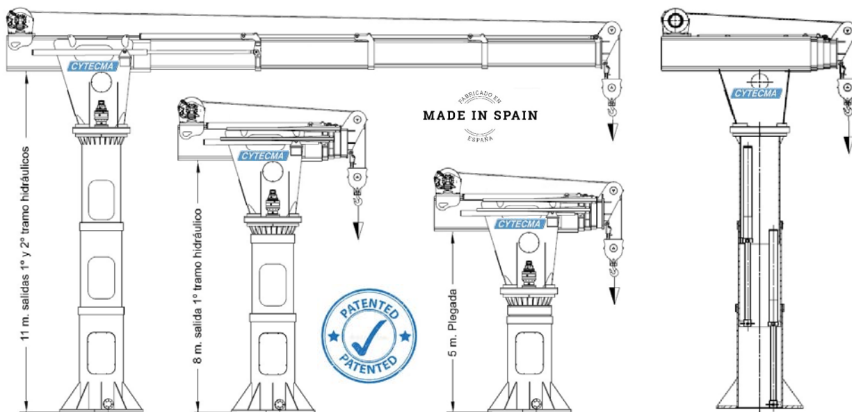
POSICIONAMIENTO HIDRAULICO DE LA ALTURA DE COLUMNA
